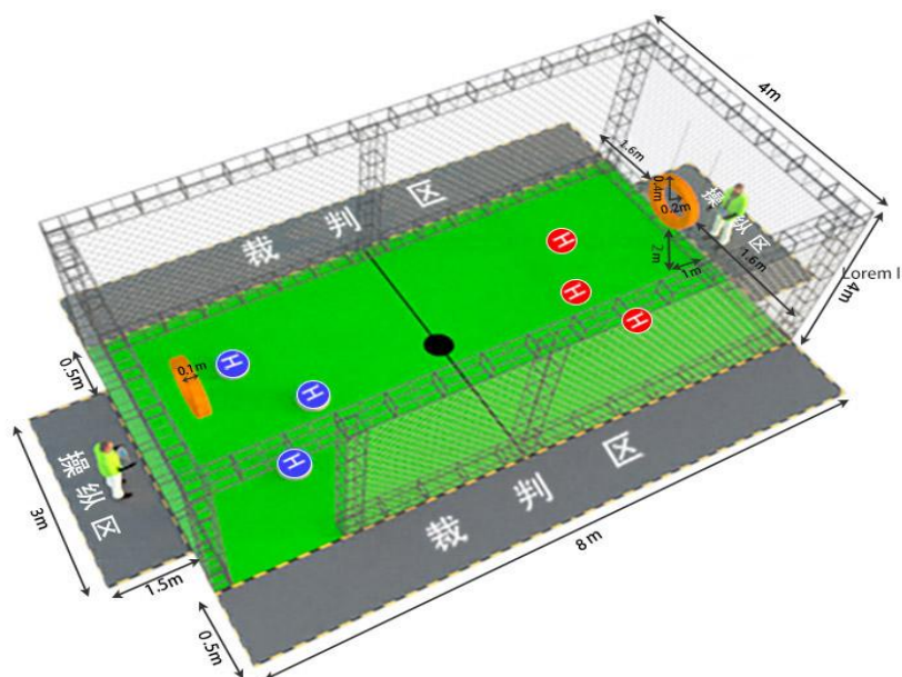
无人机足球（空心杯组）场地示意图
