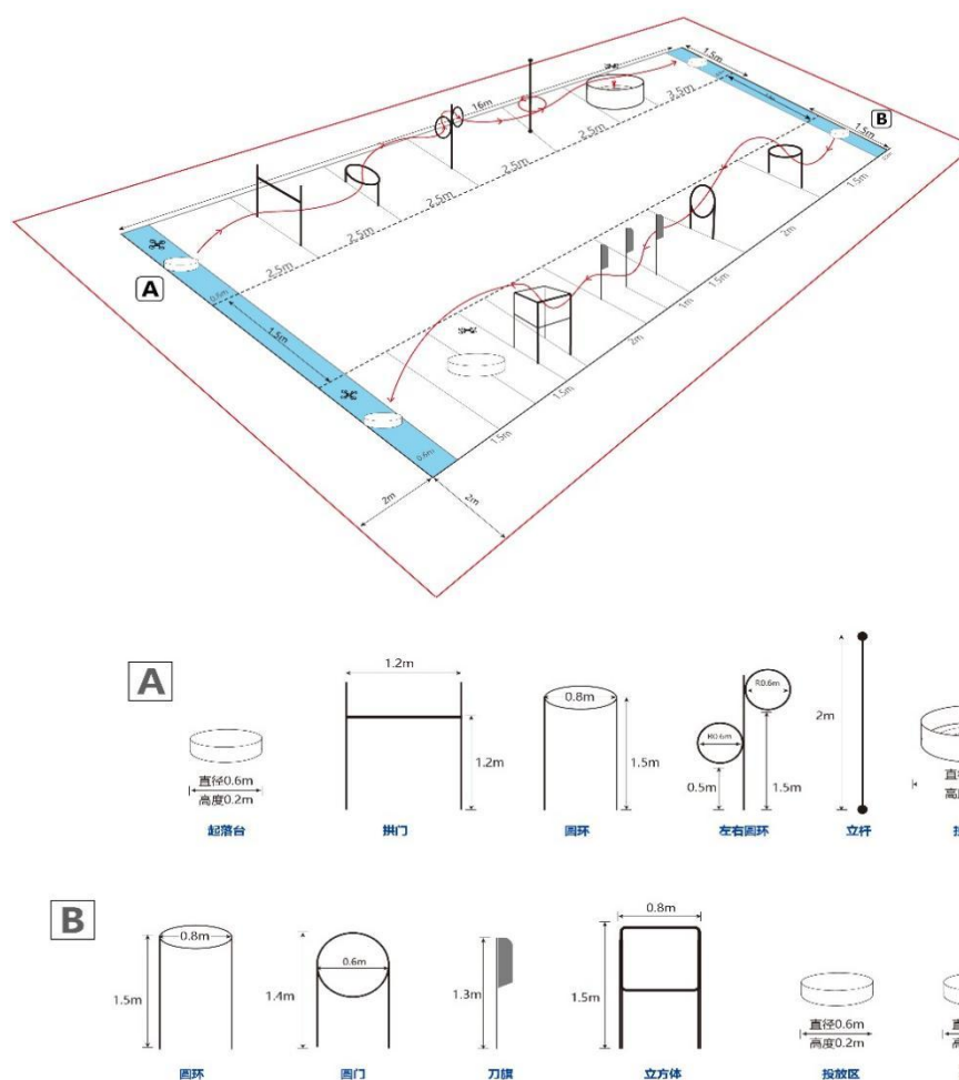
无人机运输任务场地示意图
