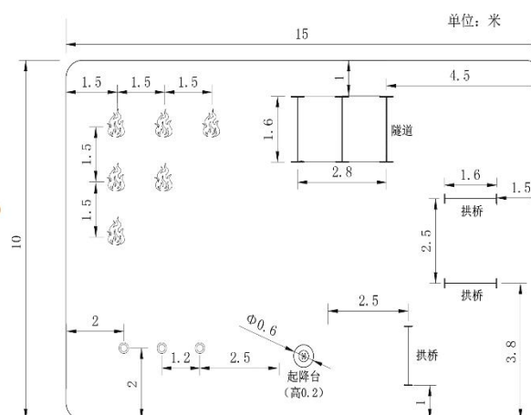
无人机灭火飞行场地示意图
